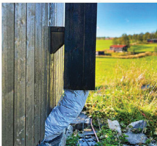
Utlufting: Vi valgte å plassere luftingen på utsiden av vegg. Da slapp vi å føre røret gjennom taket i baderommet. Selve røret ble også isolert for å unngå kondensproblemer.
