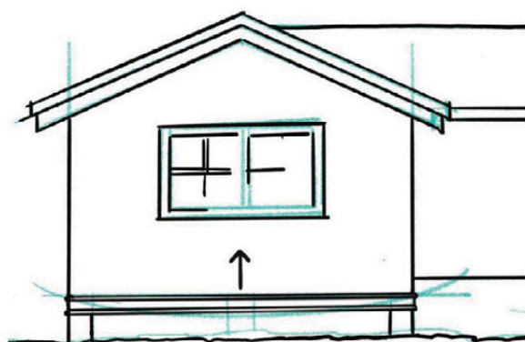
2. Bjelken ble jekket opp i hver ende.
