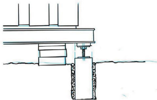
4. Når bjelken var i riktig høyde, fjernet vi jekken og støpte en pilar. Vi brukte en justerbar stolpesko for å kunne gjøre justeringer i etterkant.
