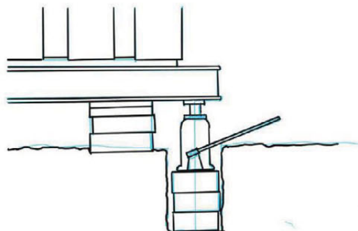
3. Biter av trevirke ble lagt både under jekken og under bjelken etter hvert som bjelken ble jekket høyere.
